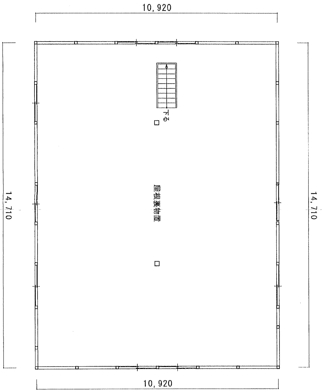
住宅2階平面図
