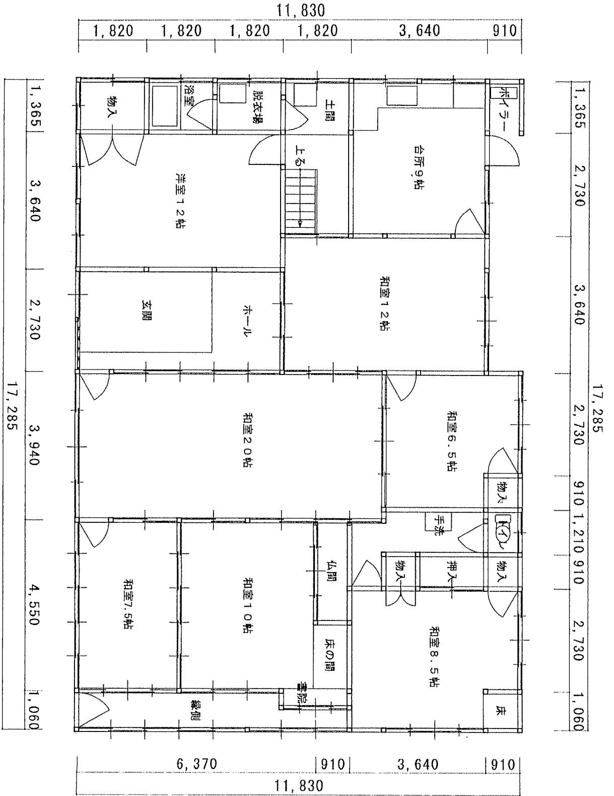
住宅 1 階平面図
