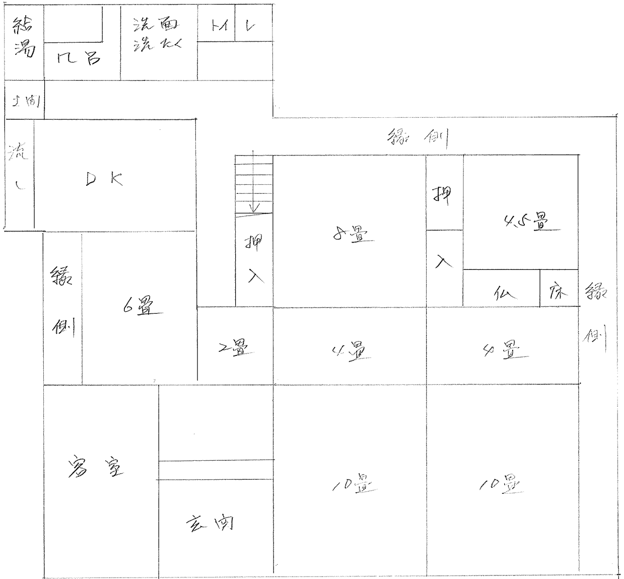
1F 平面略图
